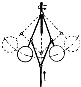
Centrifugál-regulátor
