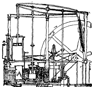
Watt gőzgépe
