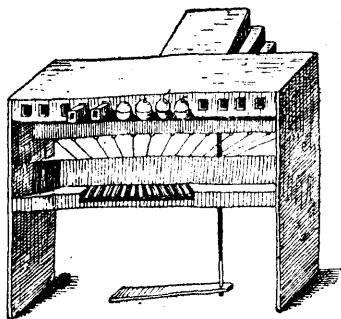
Kempelen Farkas beszélgépe
