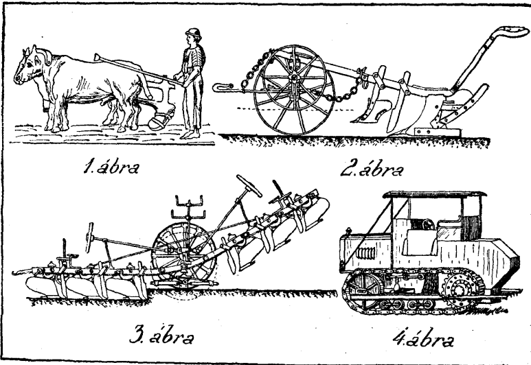
1. Etruszk eke. — 2. Modern vaseke. — 3. Háromszoros billenőke gépszántáshoz. 4. Benzinlokomobil ekevontásra, u. n. caterpillar (hernyó)
