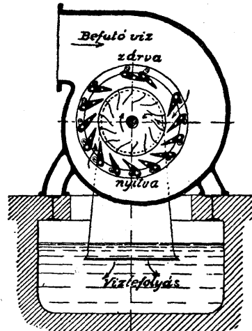
Vizturbina
