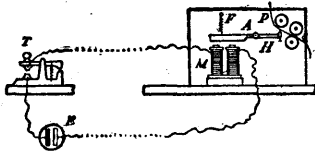
A Morse-távíró vázlatja:
