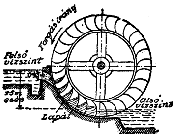
Vízikerék
