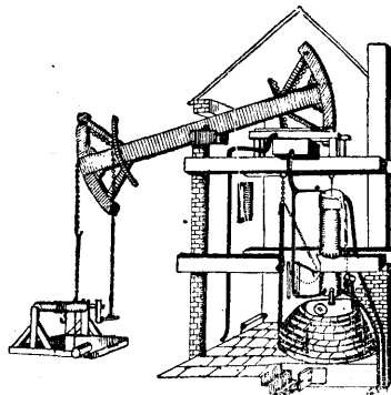
Az ujbányai régi gőzgép egykoru rajza
