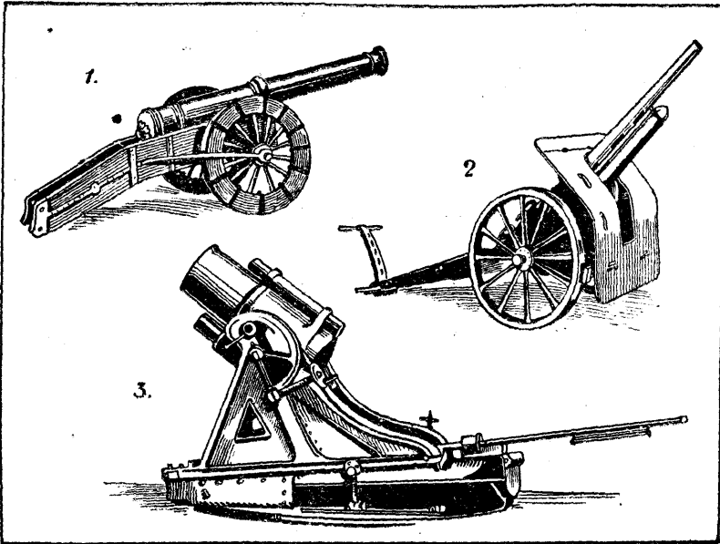
1. Német hátultöltő-ágyu 1550-ből. — 2. 7.5 cm-es Krupp-féle tábori ágyu. 3. Nehéz német aknavető.
