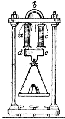
Elektromágnes: (b) vaspatkó, (a, c) tekercs, (d, e) horgony
