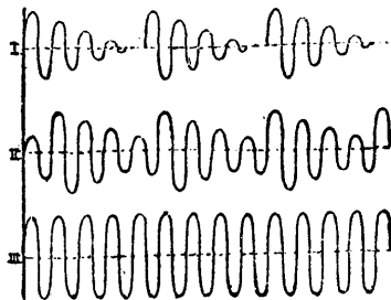
Elektromos hullámok
