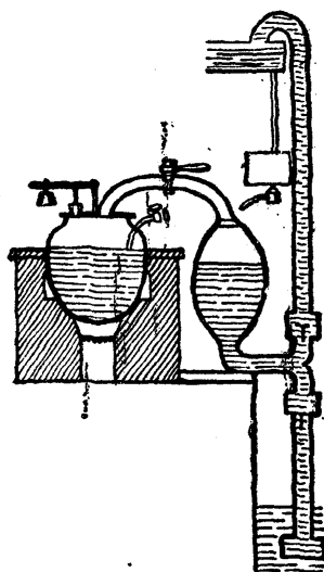
Savery aspirációs gőzgépe (1698)
