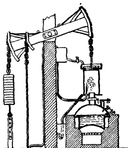
Newcomen gőzgépe (1711)
