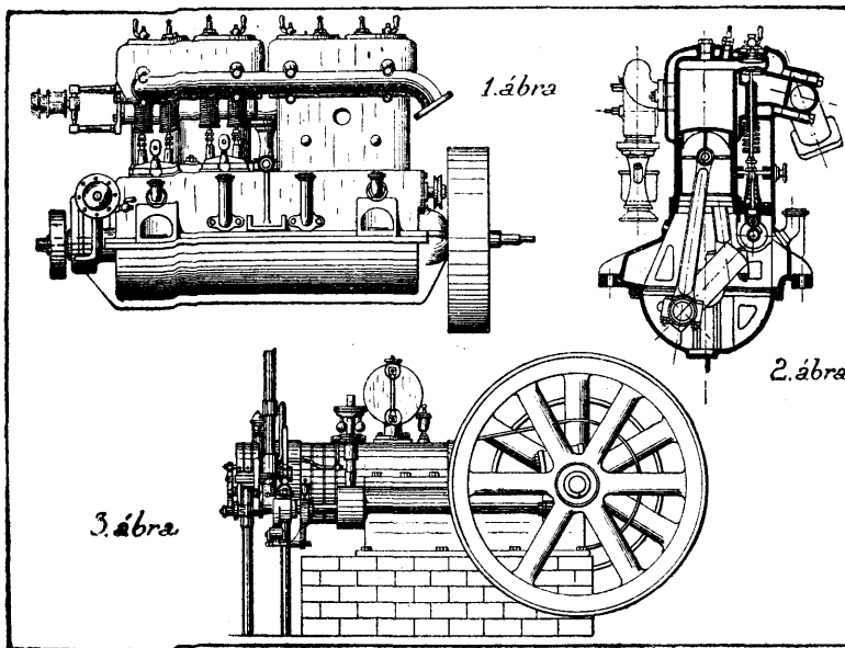
Benzin-motorok
