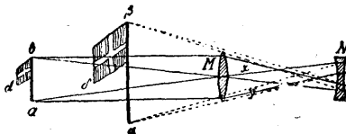
Földi távcső szerkezete
