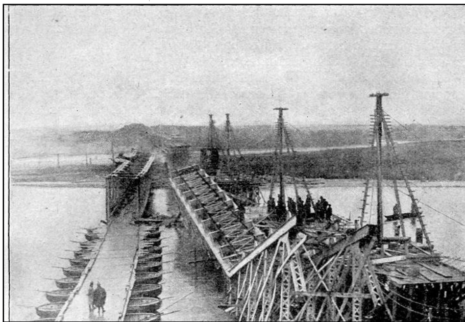
Német utászok helyreállítják a Warthán átvezető vasúti hidat a Kalina—varsói vonalon.
