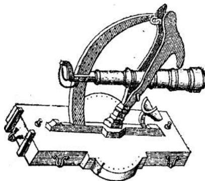
Froissart kéziratából vett ágyú.
