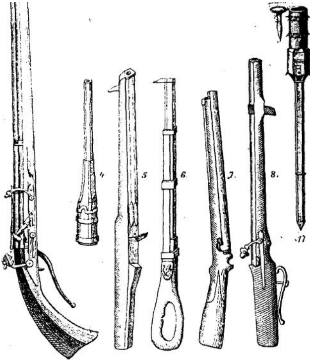
3. Kanócsos puska. 4. Kézi ágyú, 23 cm. hosszú. 5. Kézi ágyú, 35 cm. hosszú, 6. Gátpuska, 1.80 m. hosszú, a melyet Murten ostrománál Bátor Károly ellen használtak. 7. Kézi ágyú. 8. XV. századbeli haquebuse. 17: Buzogányos puska.
