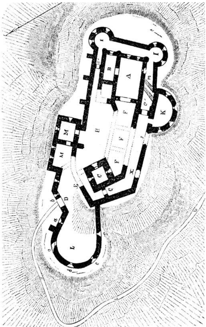
129. ábra. — A torvat vár alaprajza.
