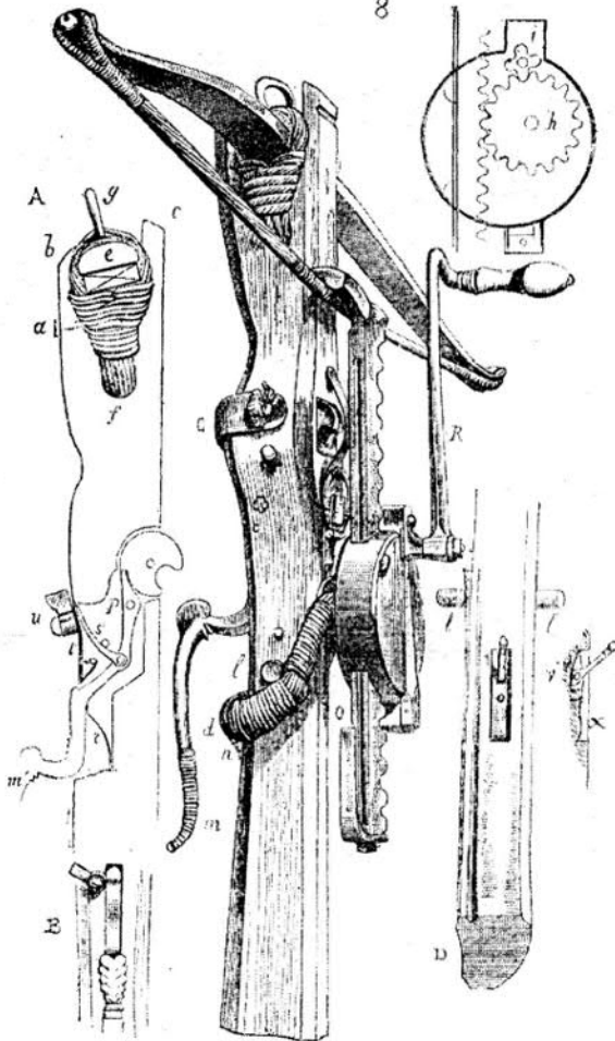
Számszerij (arb. à cric).
