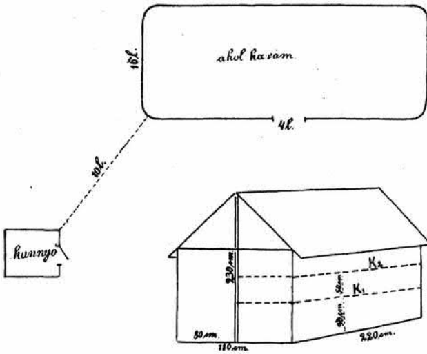
Akolkaram és nádkunyo alaprajza.
