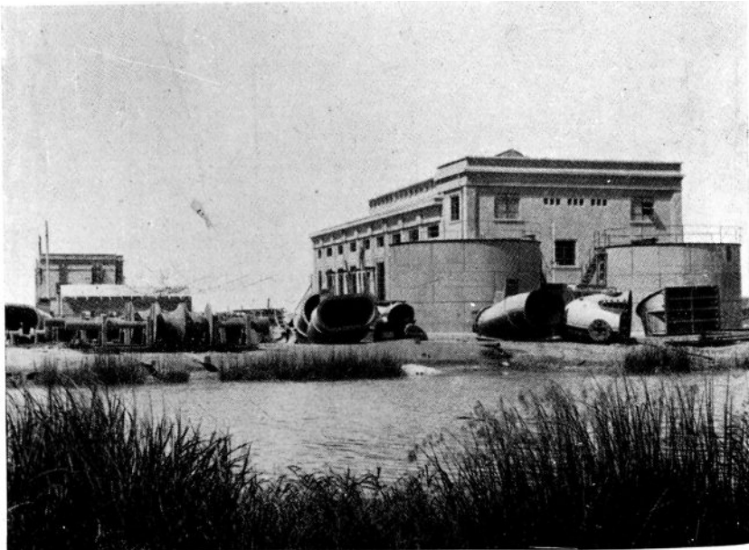
A serui lecsapoló szivattyútelep szerelés közben.
