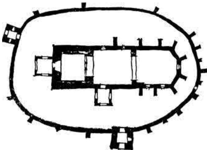
A VALKÓI (KOLOZS VÁRMEGYE) REF. KERÍTETT TEMPLOM ALAPRAJZA
