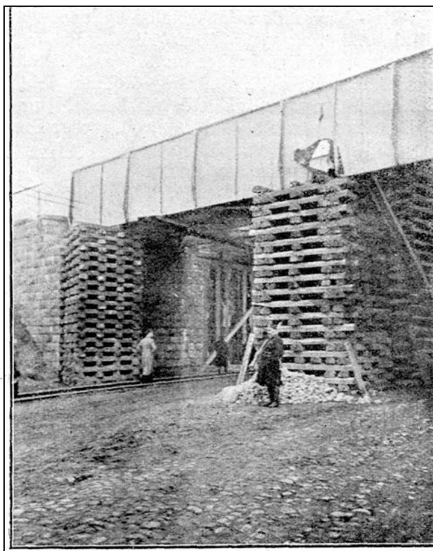
Felrobbantott és rendbehozott vasúti híd Lodzban.
