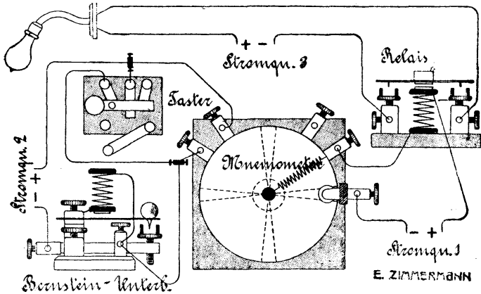
4.-ik ábra. Szabályozható, tetszésszerinti tartamú megvilágítás a Ranschburg-Focher-féle sztaniolos korong segítségével.
